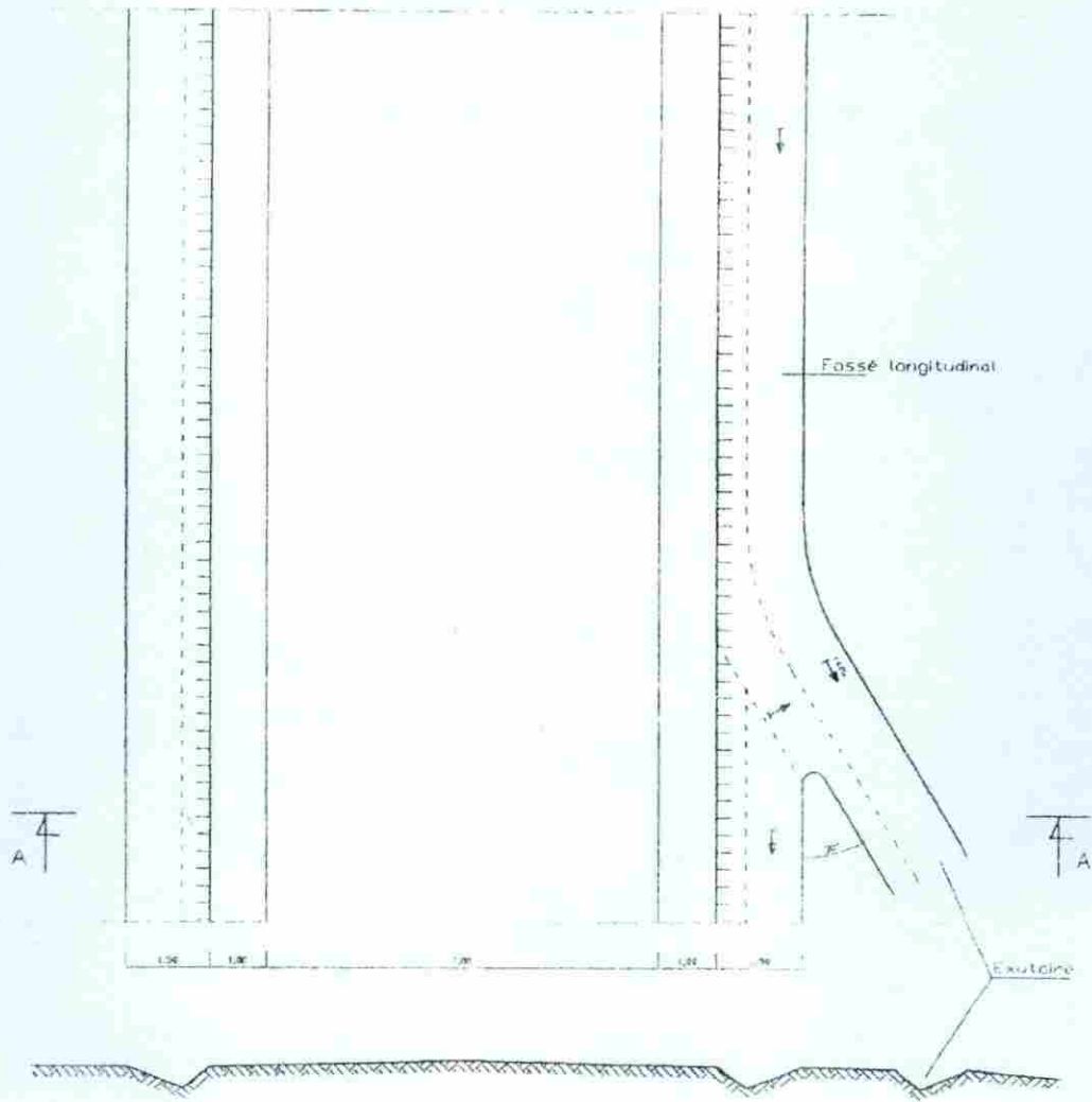
COUPE A-A
